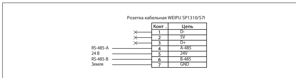
Рис.3. Схема распайки коннектора при подключении к сети электропитания 24 В и сети передачи данных на основе RS-485.
