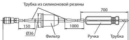
Рис.5. Пробоотборные устройства
