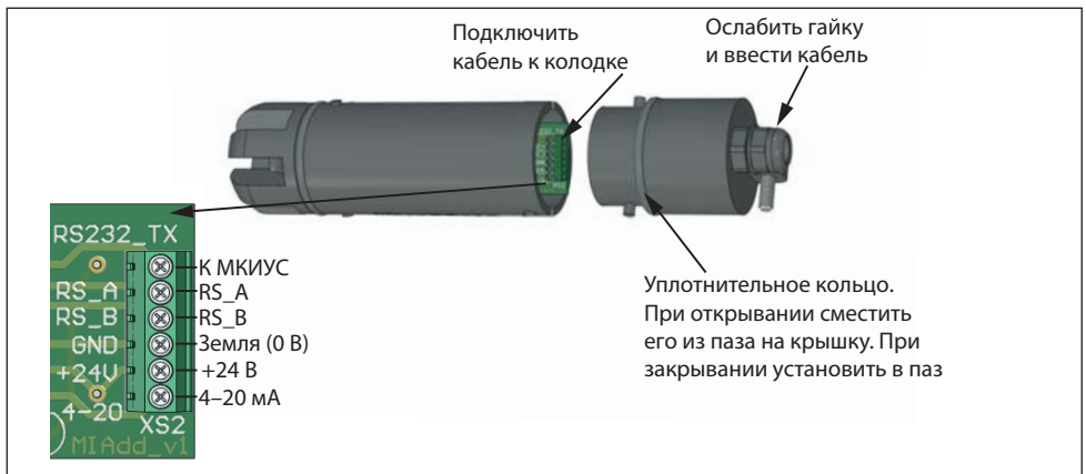
Рис.5. Порядок подключения кабеля
