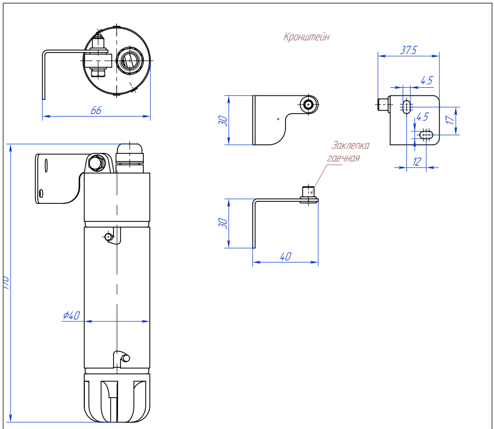
Рис.4. Габаритный чертеж "Сенсон-СД-7051"
