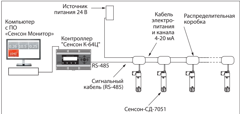
Рис.3. Основная схема подключения ГС шлейфом
