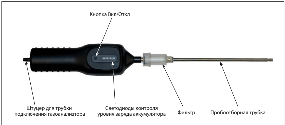
Рис. 4. Насос пробоотборный "Сенсон П-01"
