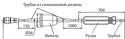
Рис.6. Пробоотборные устройства
