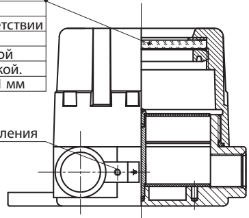
Рис.15. Элементы взрывозащиты типа "взрывонепроницаемая оболочка" модулей МКТ-3м и МКИУС
