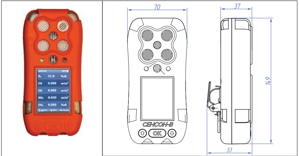
Рис. 1. Газоанализатор "Сенсон-В-4000"
