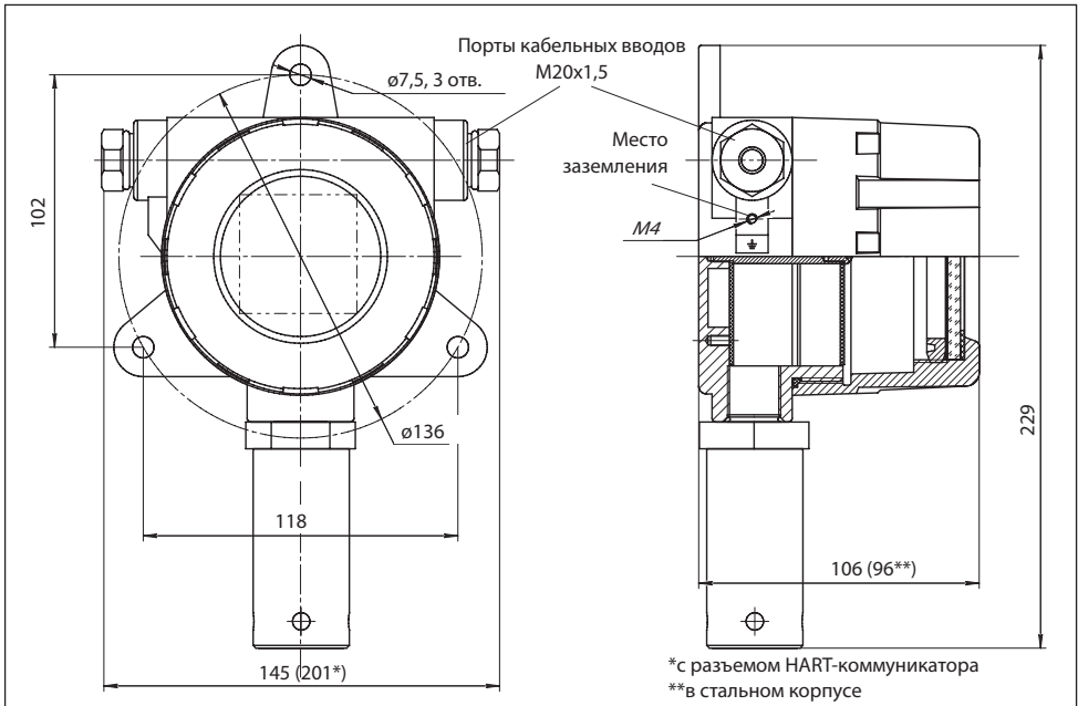
Рис.8. Габаритный чертёж ГС "Сенсон-СВ-5031-СМ"
