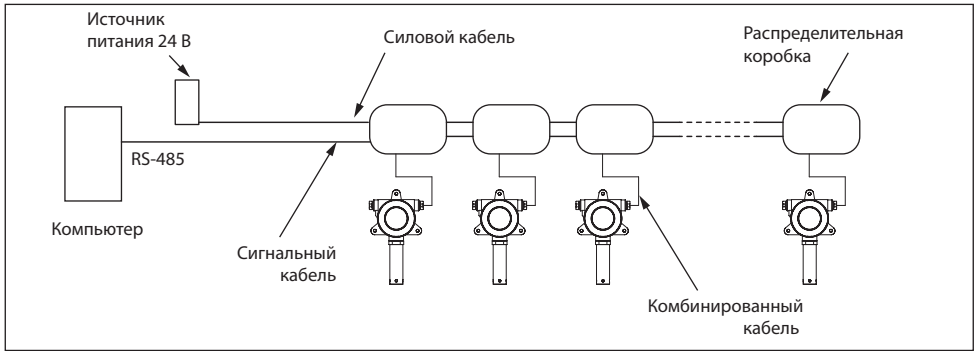
Рис.9. Схема подключения ГС шлейфом с распределительными коробками
