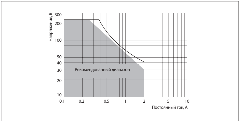
Рис.6. Допустимая мощность коммутации силовых реле
