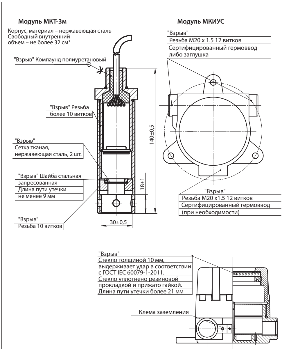
Рис.15. Элементы взрывозащиты типа "взрывонепроницаемая оболочка" модулей МКТ-3м и МКИУС
