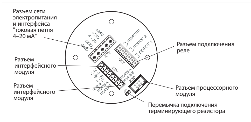
Рис.12. Модуль коммутации
