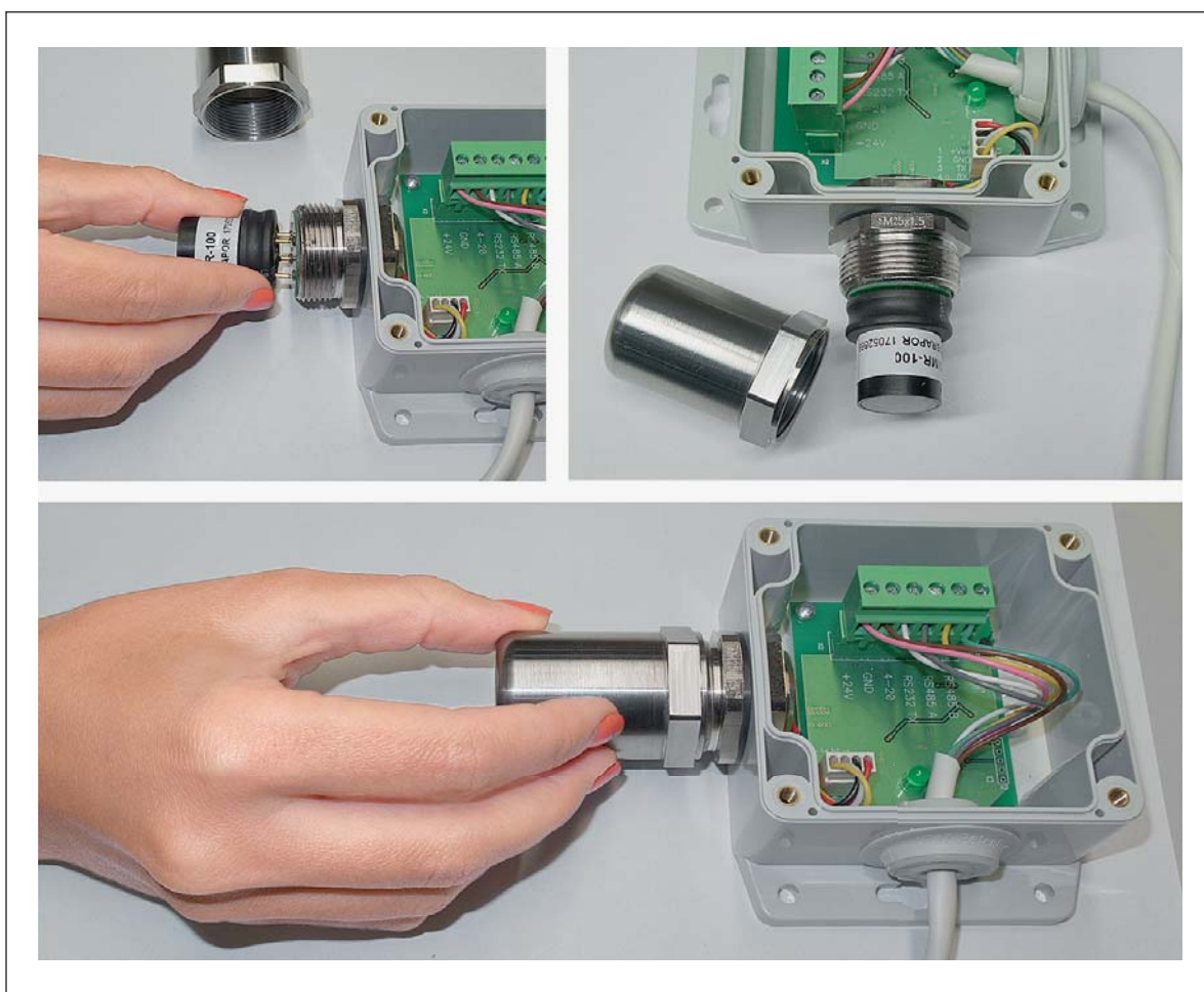
Рис.4. Установка ИСМ
